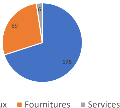
Graphique 1: Répartition des appels d'offres lancés par type
